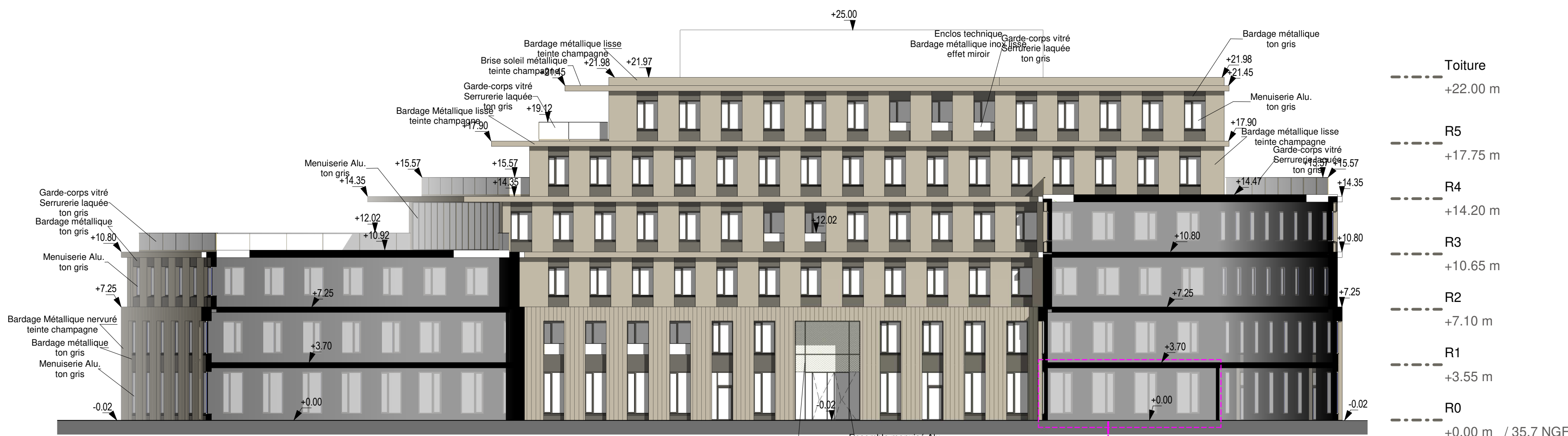
4 DS 4 : Façade - Coupe Sud 1 : 200
