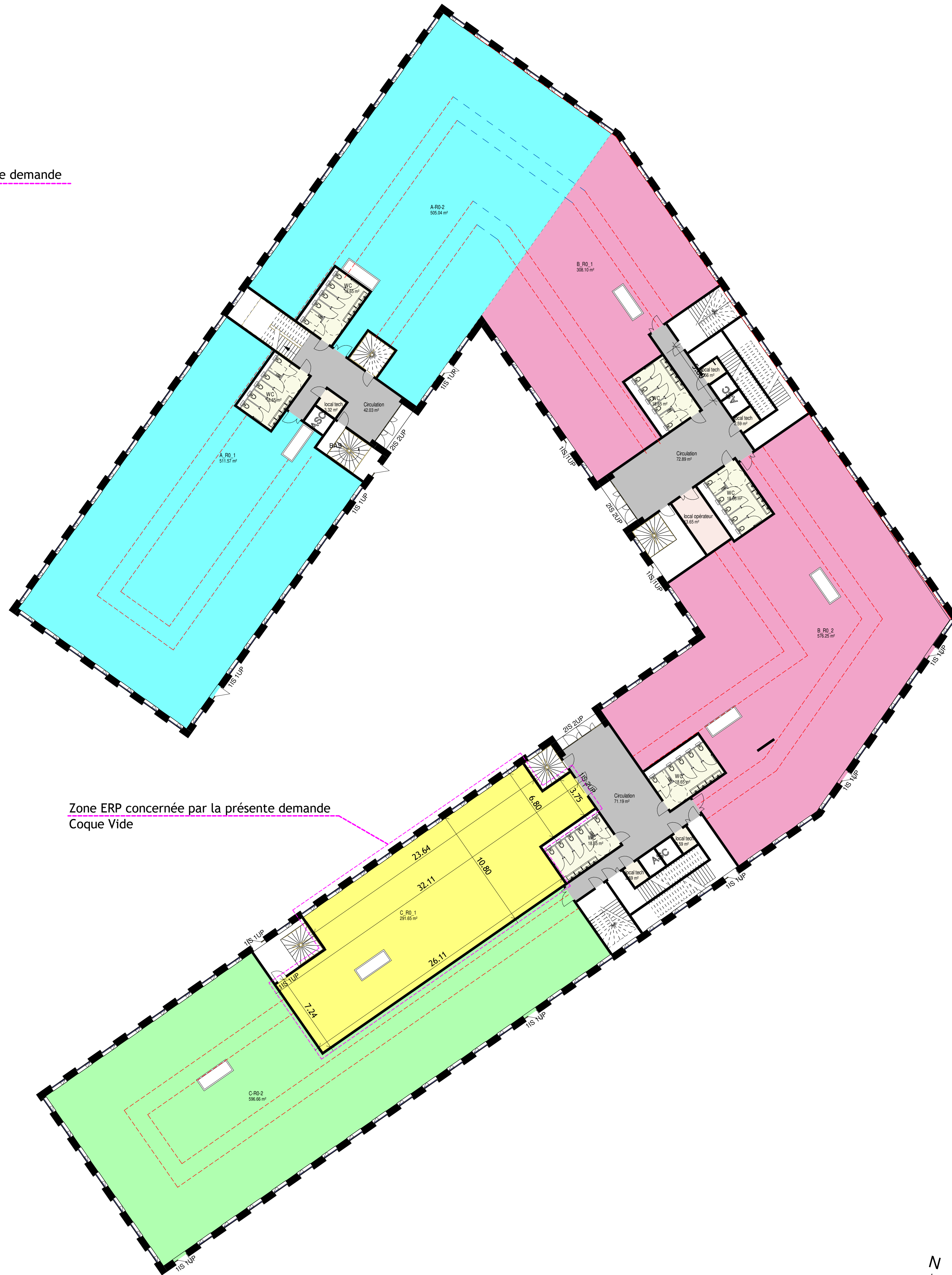
2 DS 5: Plan Rez-de-Chaussée 1 : 200
