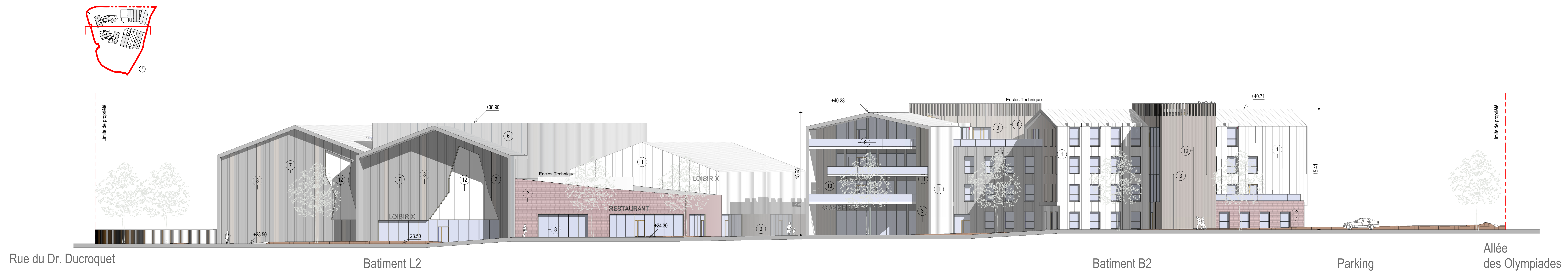
1 PC_Façade Nord Rue piétonne 1 : 200
