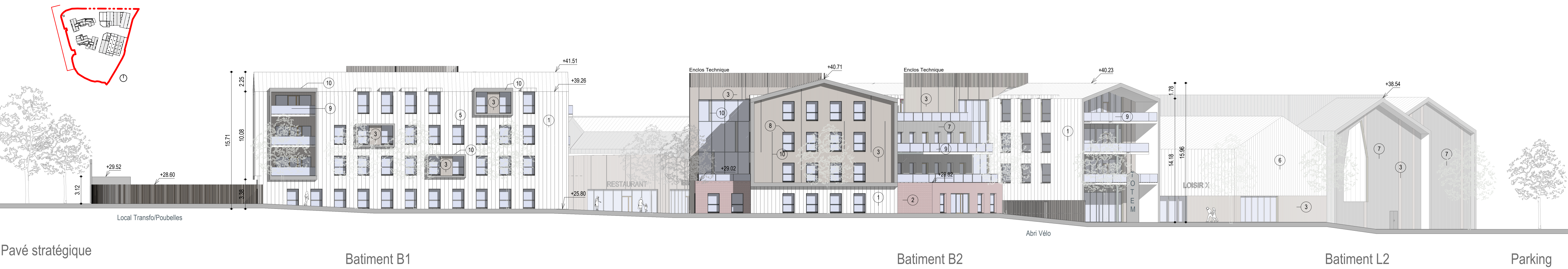
2 PC_Élévation externe Ouest 1:200
