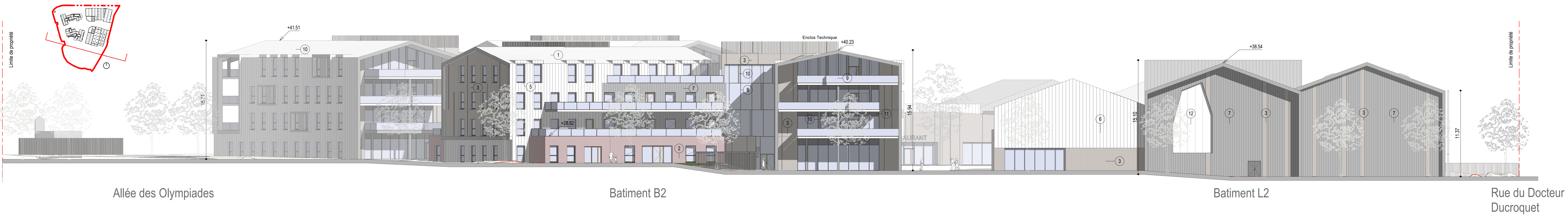
3 PC_Élévation externe Sud 1:200
