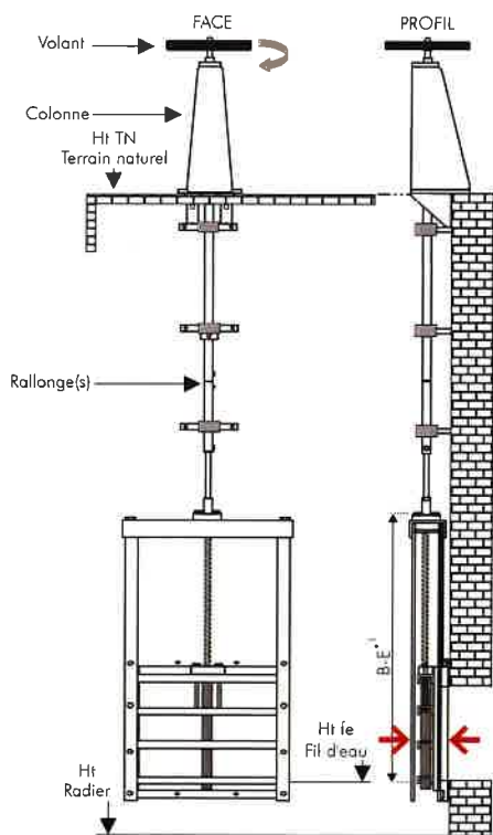
MODÈLE 3 : Vanne + Rallonge(s) + Colonne inclinée + Volant.
