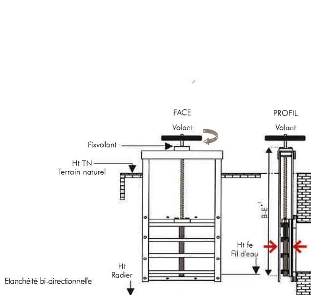
MODÈLE 2 : Vanne + Fixvolant + Volant
