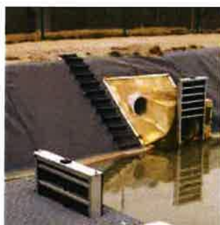
Déversoir rotatif
