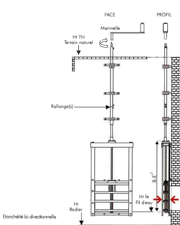
MODÈLE 4 : Vanne + Rallonge(s) dépassant niveau TN + Manivelle (ou clé en T, la connexion en extrémité supérieure de la rallonge est au niveau du TN).
