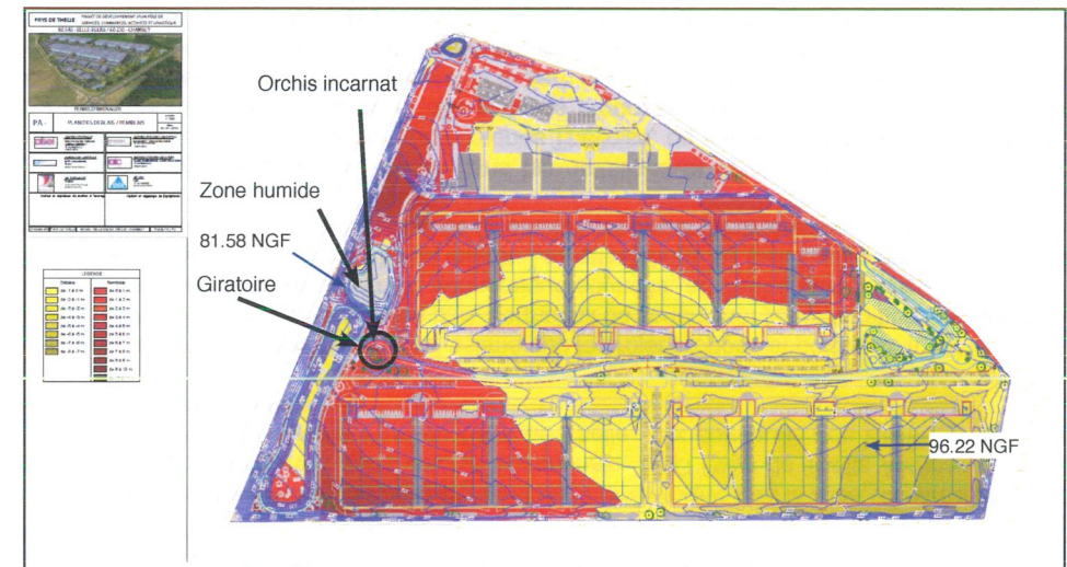
Plan du déblais-remblai du site de projet
