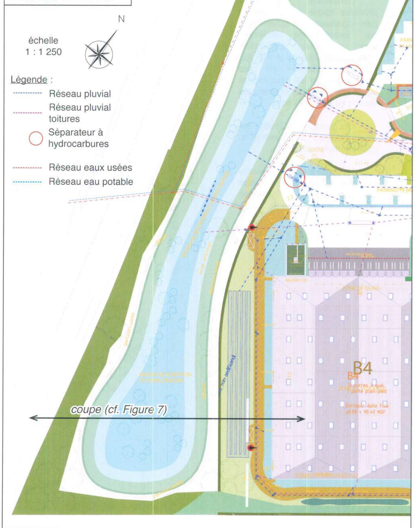
FIGURE 8 : PARTIE PARC LOGISTIQUE : ZOOM SUR LE BASSIN D'INFILTRATION
