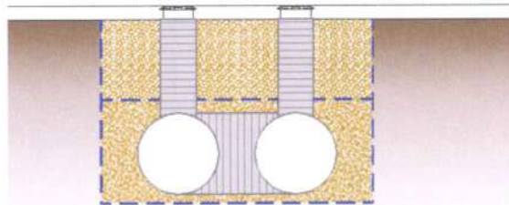
Coupe du réservoir sous le niveau du sous-sol
