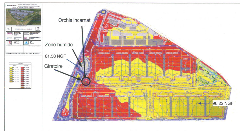
Plan du déblais-remblai du site de projet
