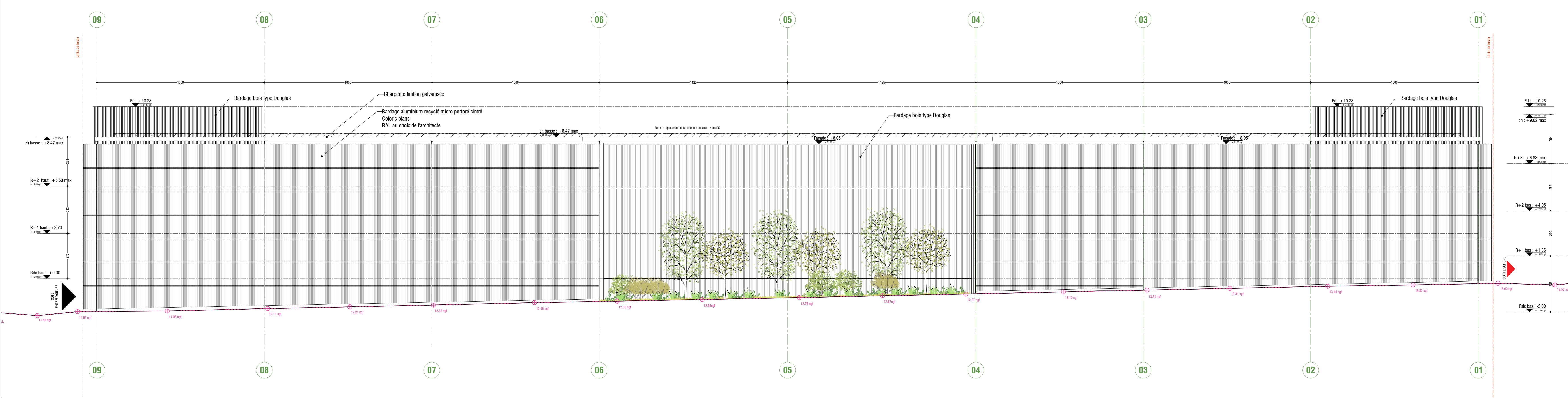
Elévation Est
