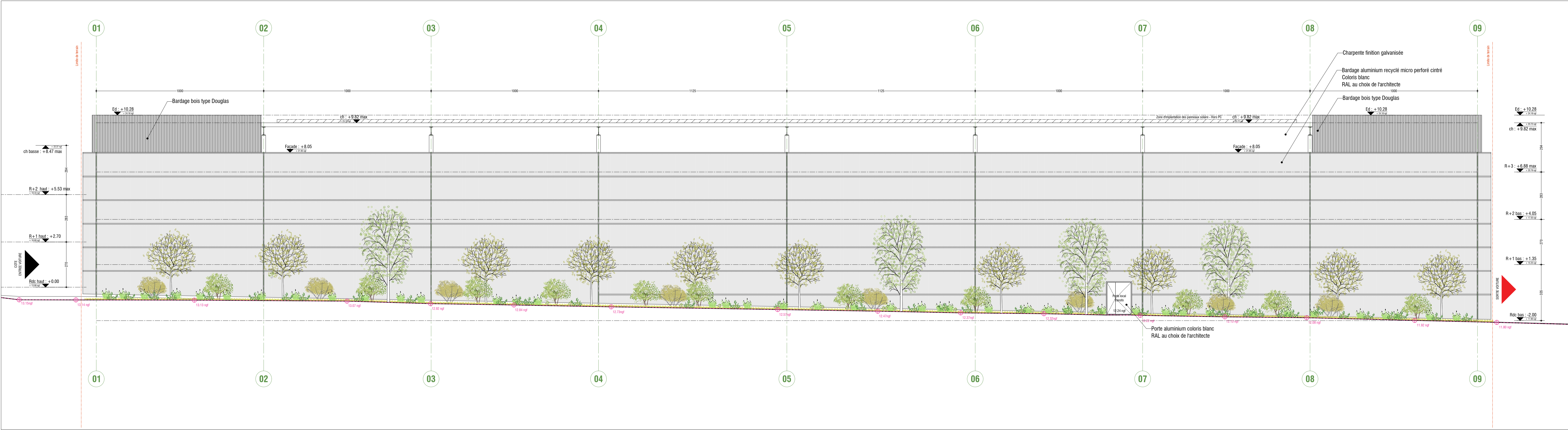
Elévation Ouest
