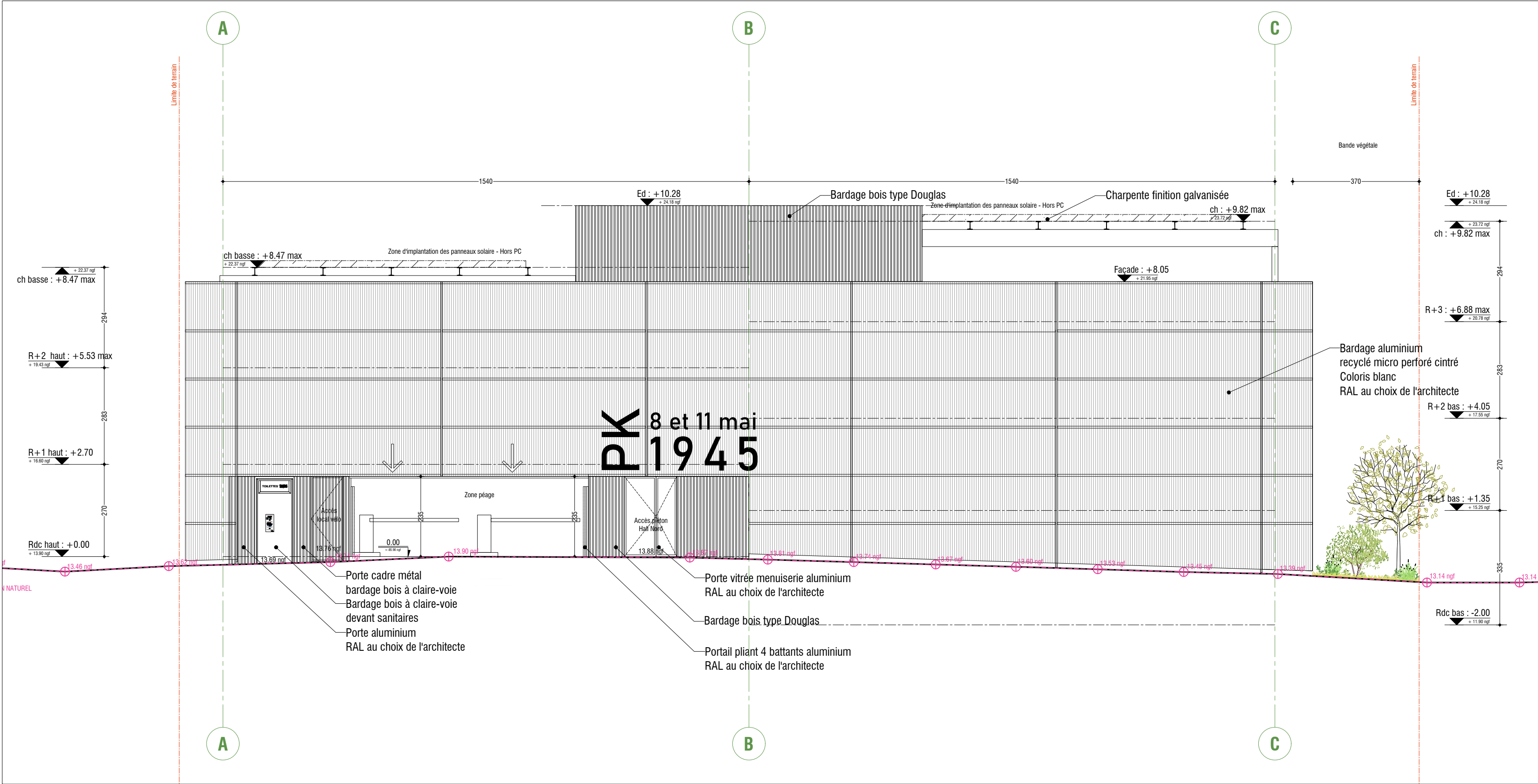
Elévation Nord
