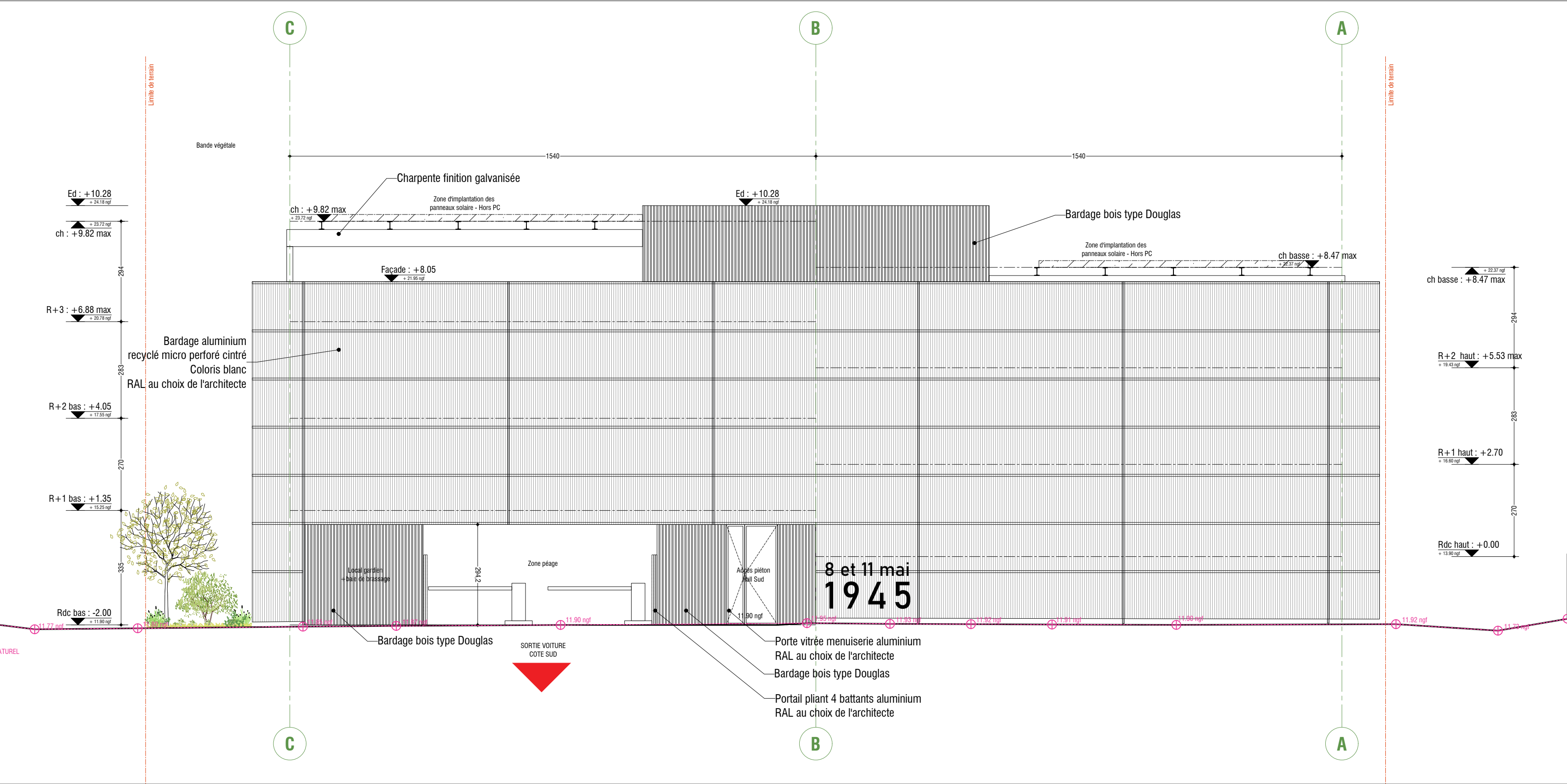
Elévation Sud
