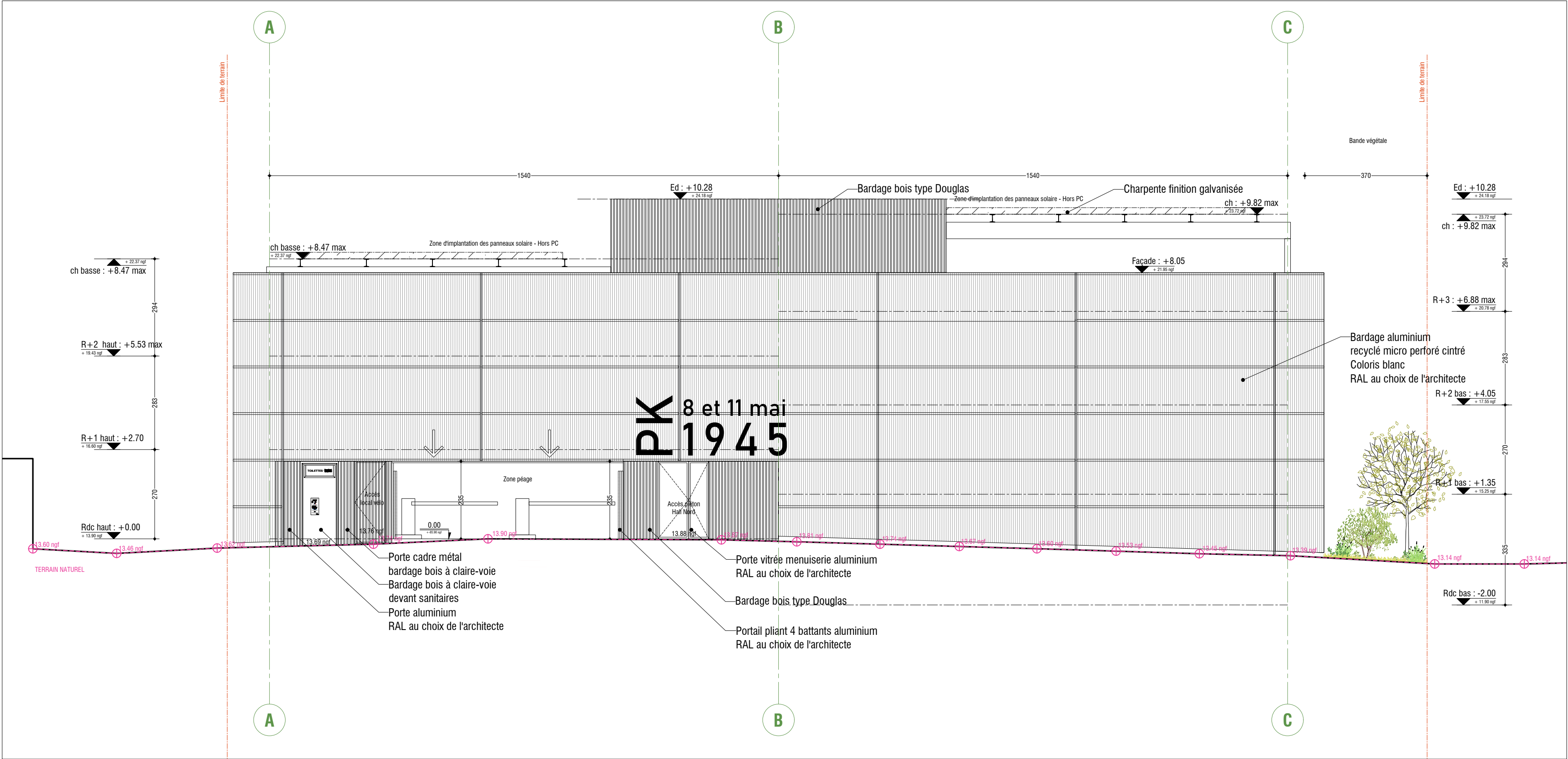
Elévation Nord
