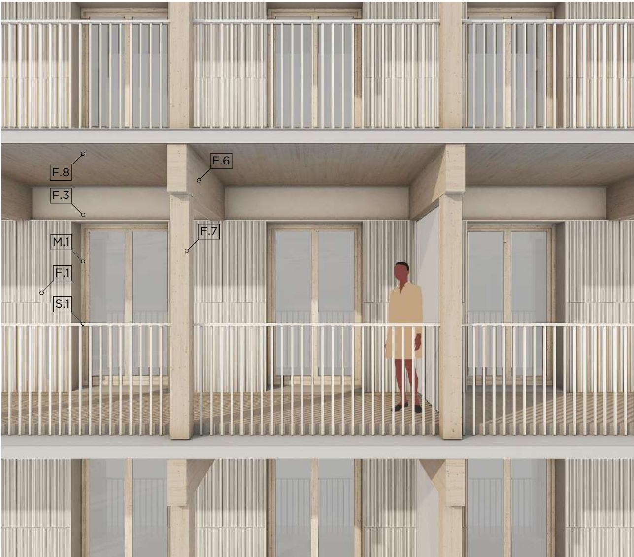
Légende (dito PC5) de façade avec loggias (R+5+6+7+8) surélevée (S-E)
