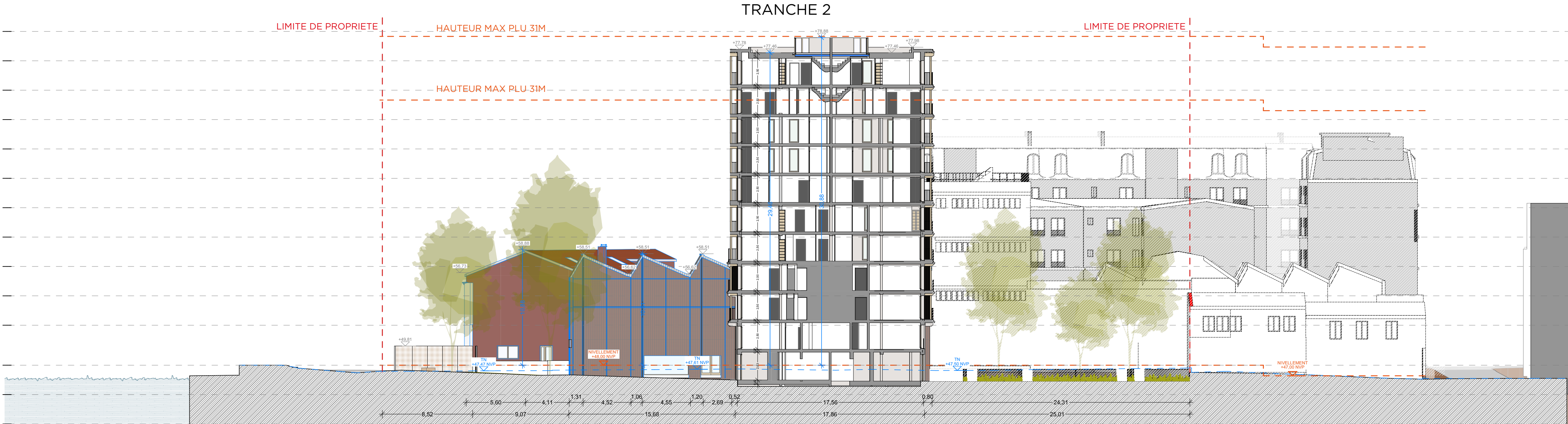
COUPE FACADE CC' FACADE NORD EST DES PLOTS C, D, E ET F
