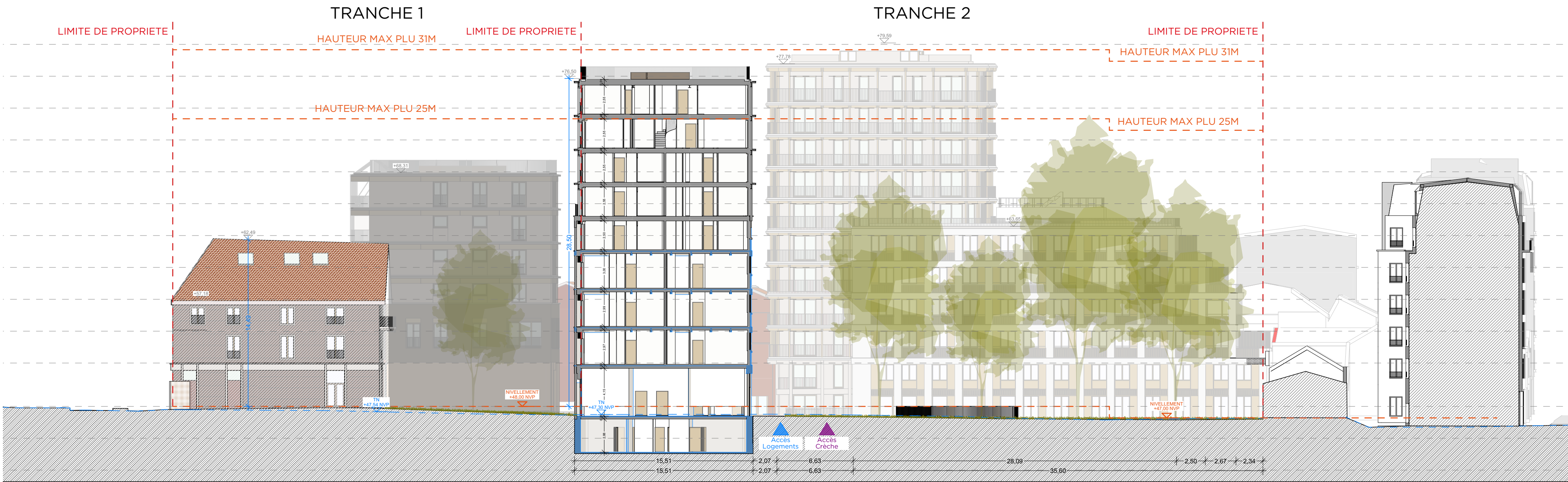
COUPE FACADE BB' FACADE SUD EST DE LA TRANCHE 1 ET DES PLOT B ET F
