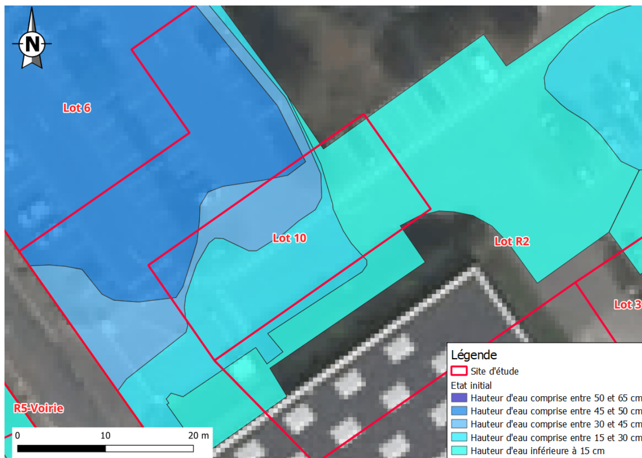
Figure 14 : Maillage par cotes altimétriques homogènes du Lot 10 à l'état initial (Source : BNP PARIBAS REAL ESTATE, sur fond de plan géoportail)
