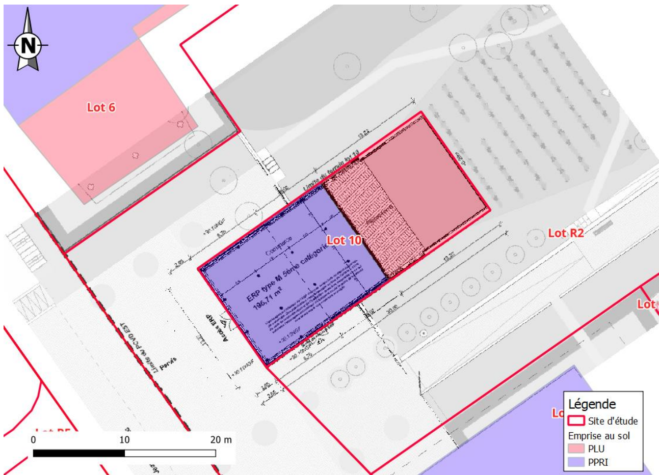
Figure 16 : Emprise au sol du Lot 10 (Plan : Rez-de-Chaussée, DGM mai 2024)
