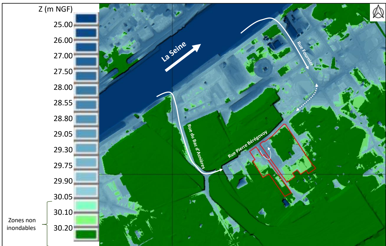
Figure 7 : Mécanisme d'inondation du site (Source : IGN, RGE Alti 1m)
