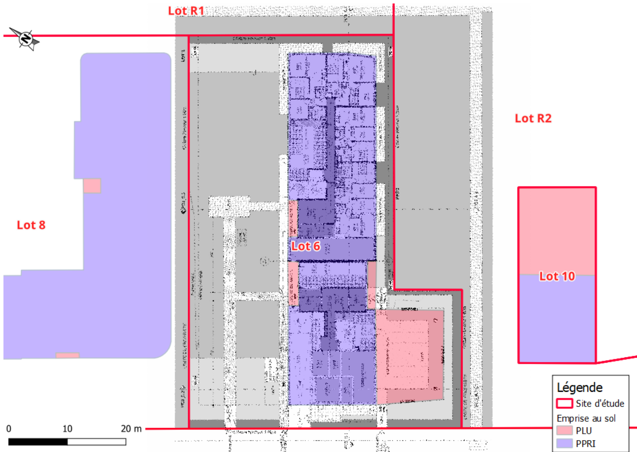
Figure 16 : Emprise au sol du Lot 6 (Plan : Rez-de-Chaussée, SNØHETTA Studio Paris, avril 2024)
