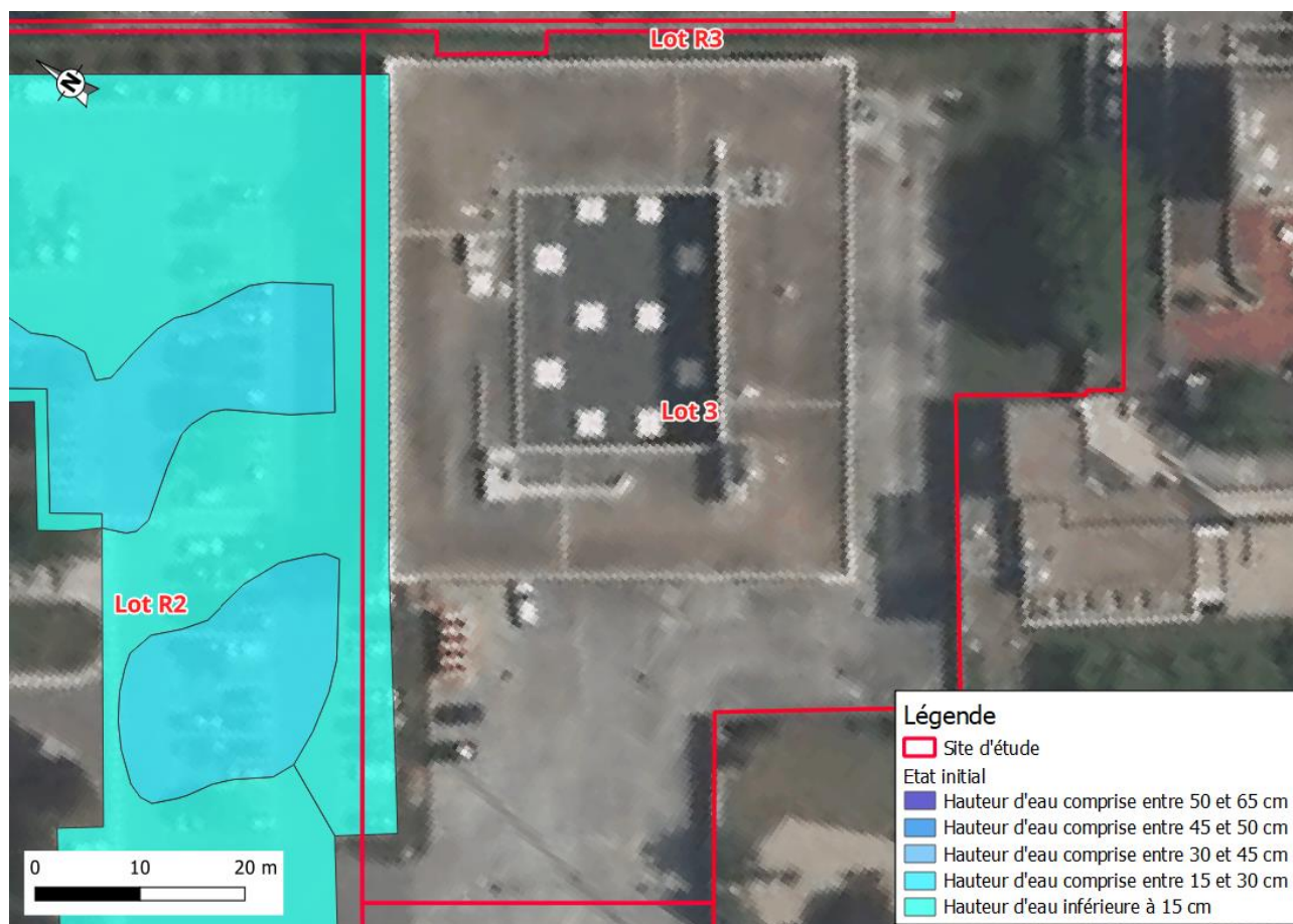
Figure 14 : Maillage par cotes altimétriques homogènes du Lot 3 à l'état initial (Source : BNP PARIBAS REAL ESTATE, sur fond de plan géoportail)
