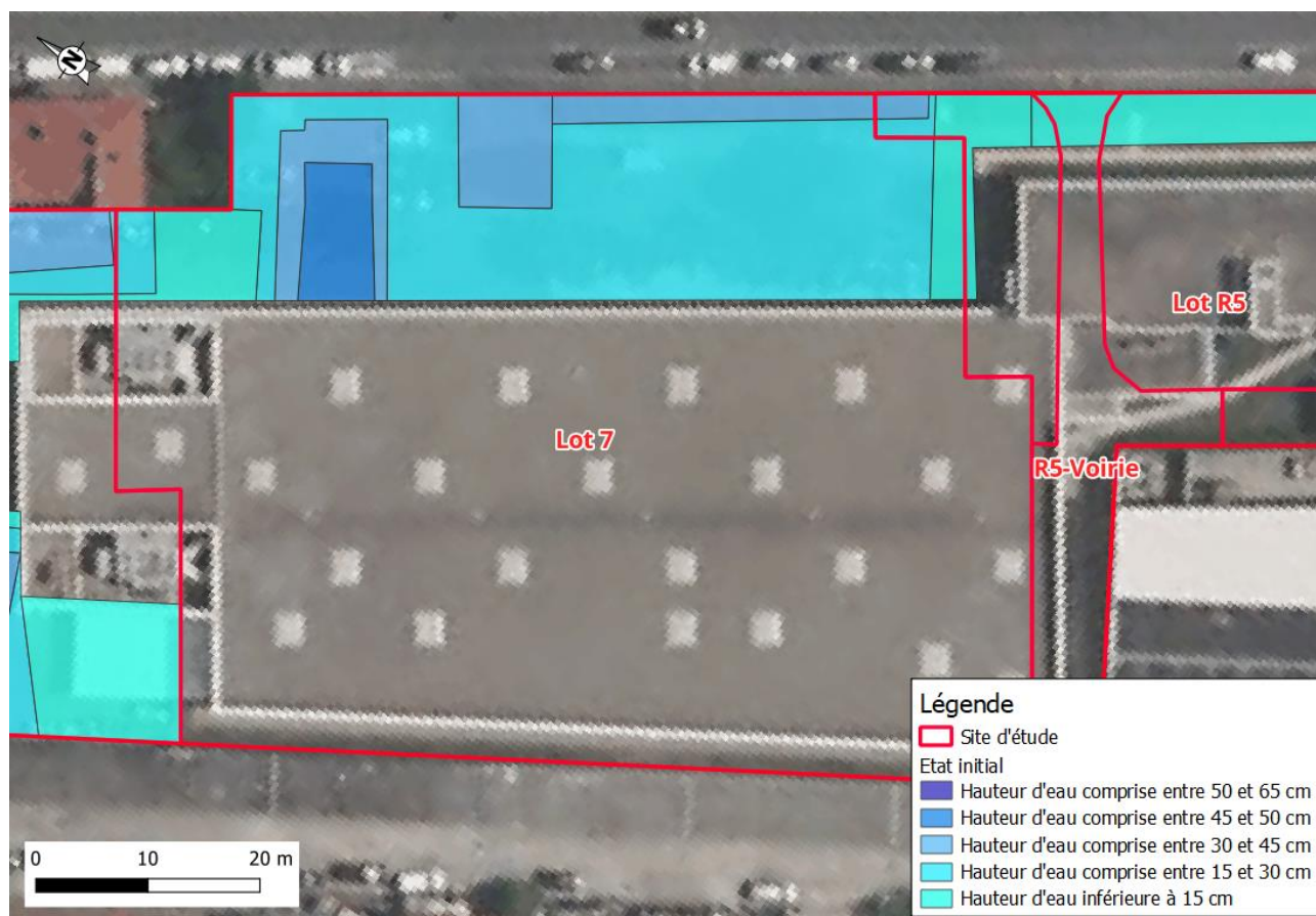
Figure 14 : Maillage par cotes altimétriques homogènes du Lot 7 à l'état initial (Source : BNP PARIBAS REAL ESTATE, sur fond de plan géoportail)
