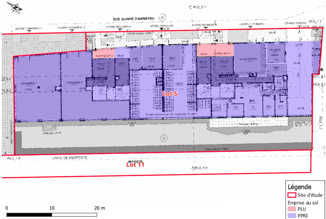
Figure 16 : Emprise au sol du Lot 5 (Plan : Rez-de-Chaussée, SNØHETTA Studio Paris, avril 2024)
