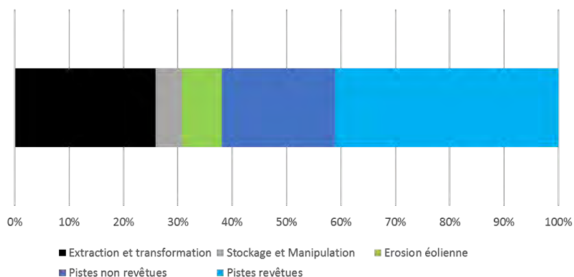
Figure 16 : Répartition des émissions de PM10 des principales sources d'émissions d'une carrière
