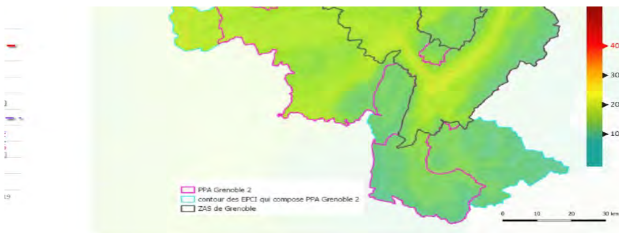
Figure 58 : Concentrations annuelles en PM 10 en 2017 (Source : Atmo AURA)
