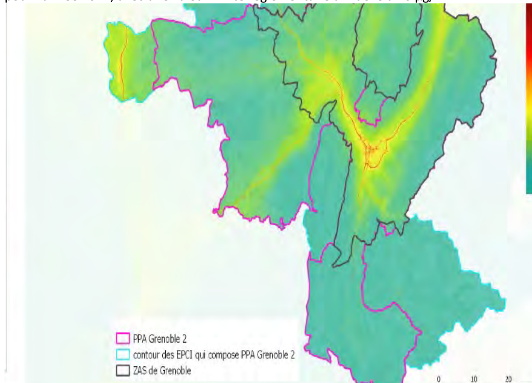
Figure 55 : Concentrations annuelles en NO 2 en 2017 (Source : Atmo AURA)
