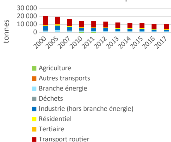
Evolution des émissions de NOx par secteur
