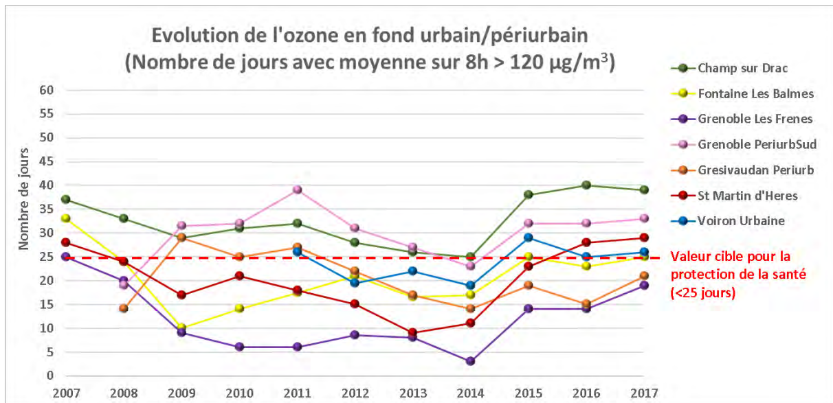
Figure 63 : Historique des moyennes annuelles en ozone à situation de fond urbain et périurbain (Source : Atmo AURA)
