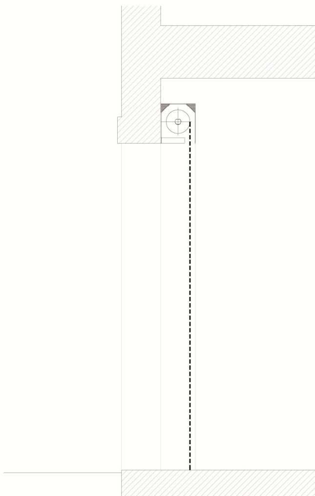
Implantation acceptable des volets roulants
