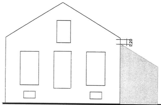
Pavillon sans escalier latéral : cas de l'extension couverte à une pente
