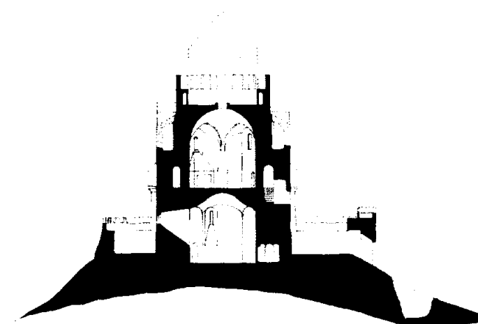
Phase 1- Plan et Coupe suivant AA
