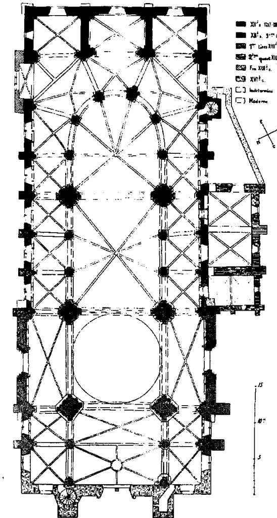
FIG. 12. — SAINT-QUIRICE. Plan dressé par F. Sautet et teinté par A. de Maillé.
