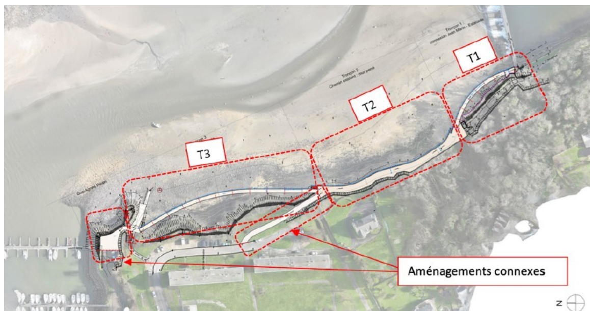
Plan masse du projet (source : étude d'impact)
