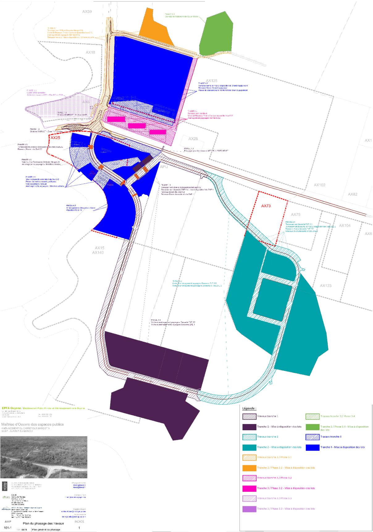
Figure 2 - Plan de phasage général des travaux
