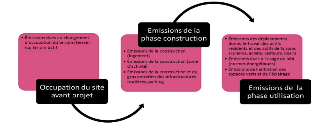
Figure 5 - Principales sources d’émissions par phase d’un projet d’aménagement
