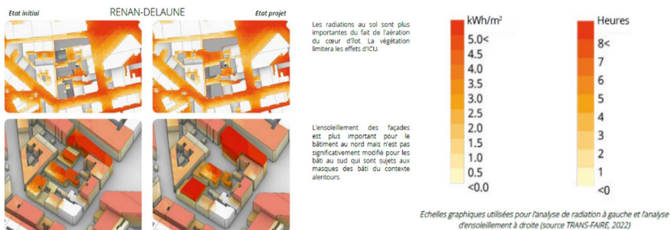
Figure 11: Extrait de comparaison des analyses de radiation (à gauche) et d'ensoleillement des façades (à droite) à l'état initial et à l'état projet, sur l'îlot « Renan-Delaune », étude d'impact (p. 246)
