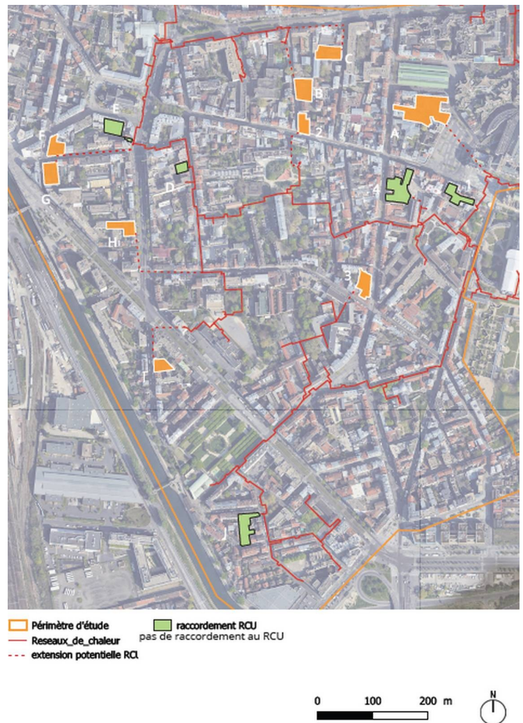
Figure 10: Réseau de chaleur et localisation des opérations potentiellement raccordées en vert (étude EnR&R, p. 22)
