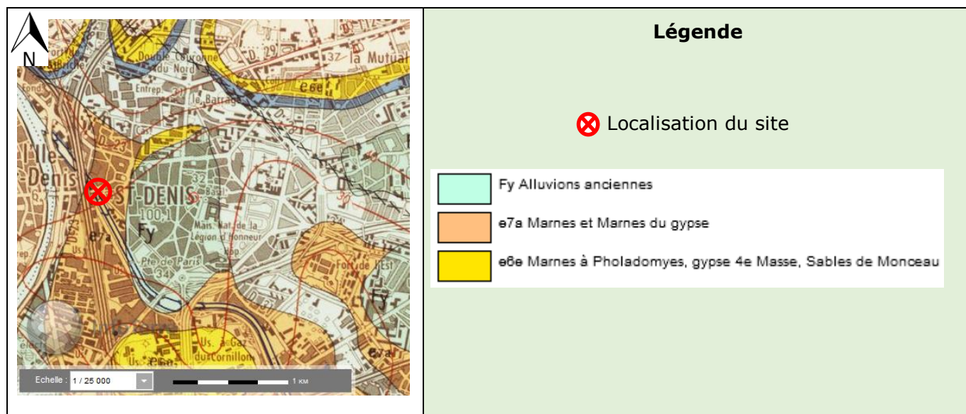
Figure 6 : Extrait de la carte géologique de PARIS au 1/25 000 ème du BRGM (source : Infoterre)
