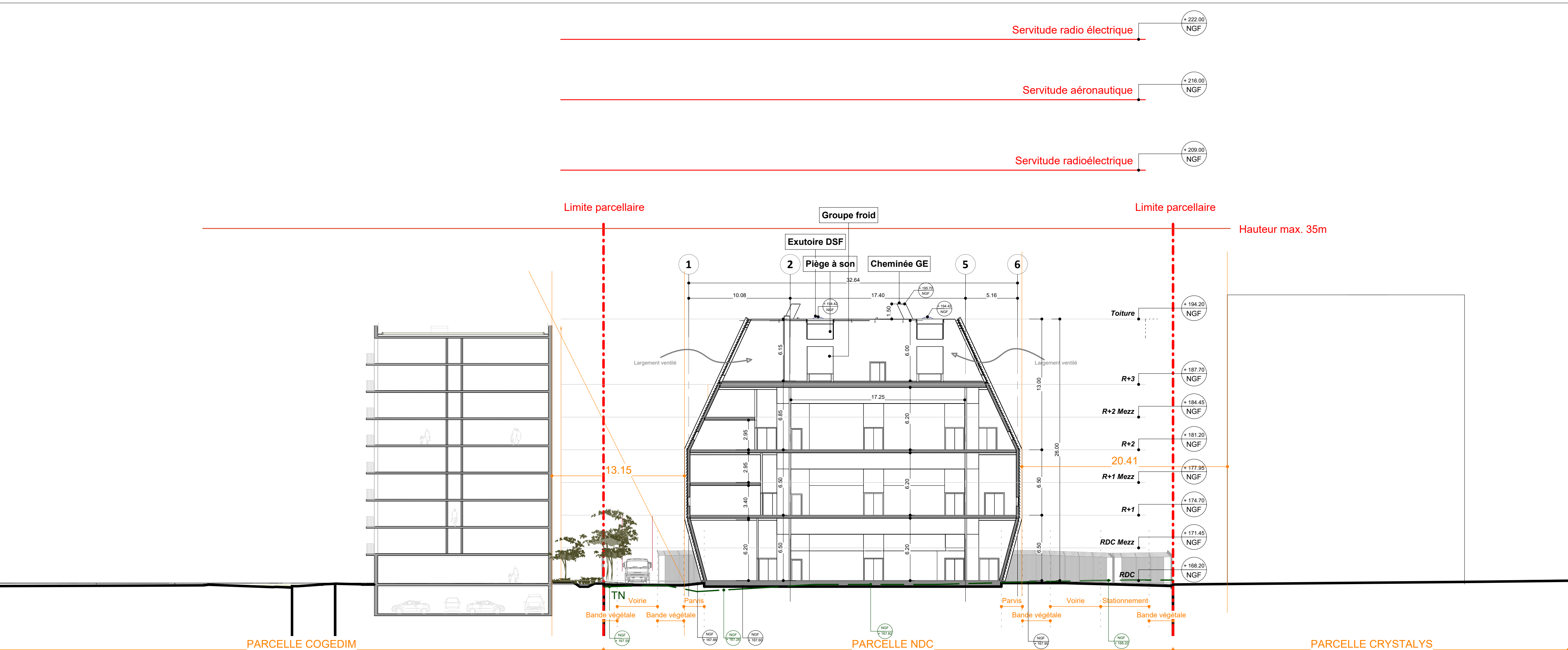
c B - Data center - Coupe transversale Ech : 1 : 250
