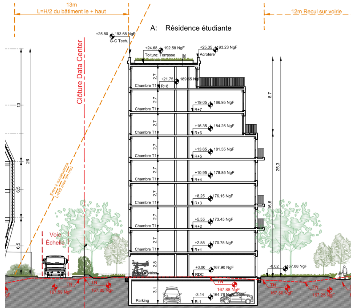
Coupe transversale du bâtiment « résidence étudiants sociale »
