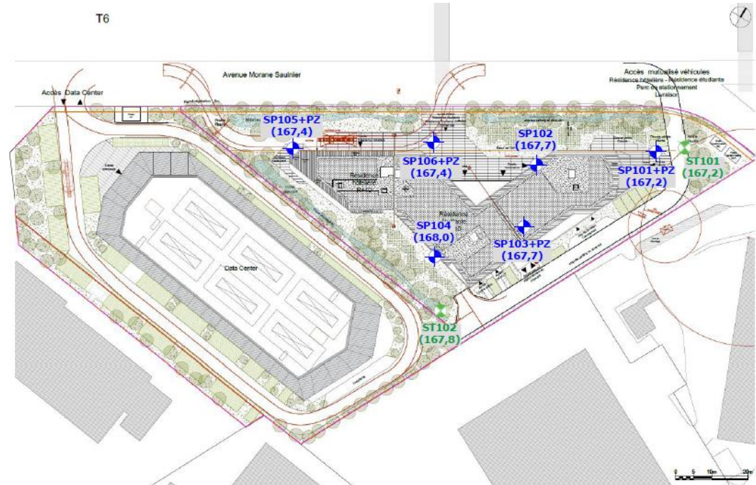
Plan de localisation des sondages (partie « résidence »)
