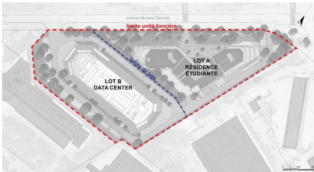
Plan de masse des lots
