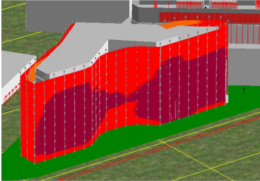
Modélisation 3D des niveaux de bruit par étage sur la façade Nord
