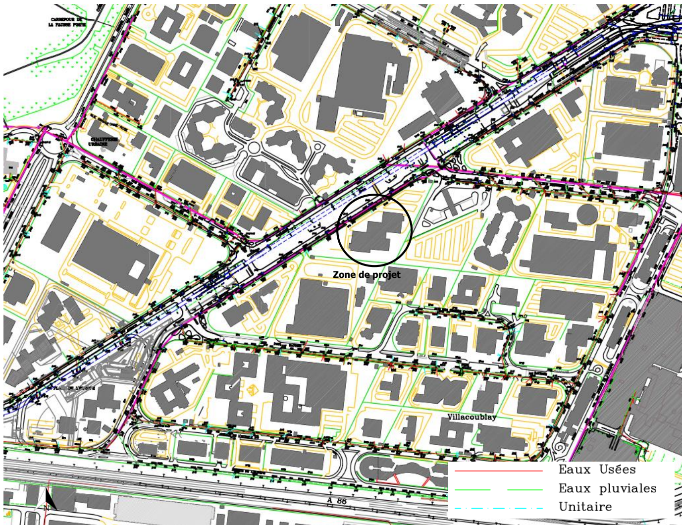
Réseau d'eaux usées et eaux pluviales à l'échelle du secteur et au droit du site de projet
