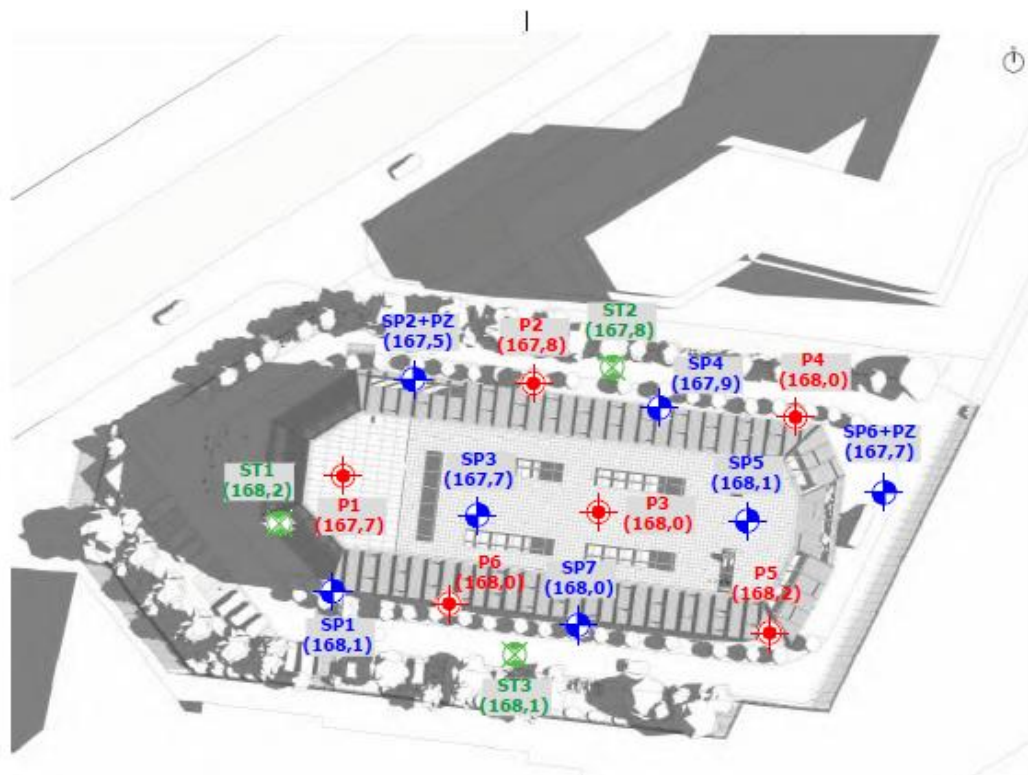
Plan de localisation des sondages (partie « data center »)
