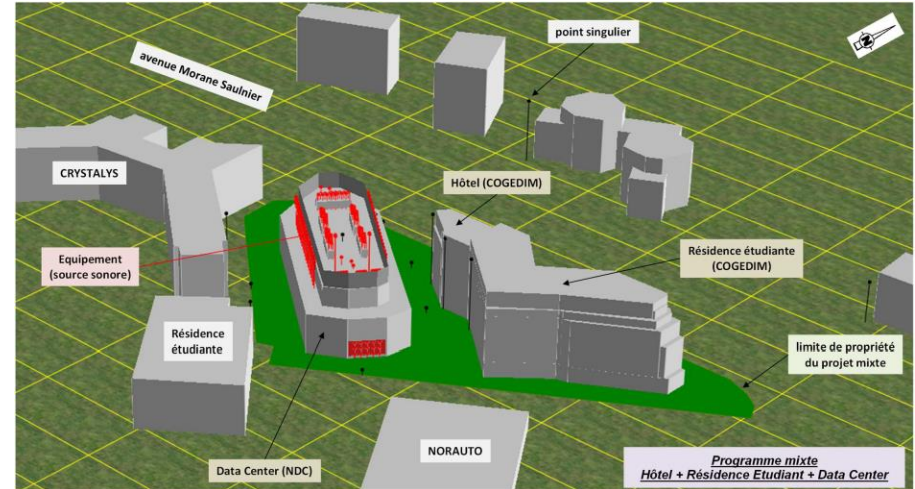
Modélisation informatique 3D du projet
