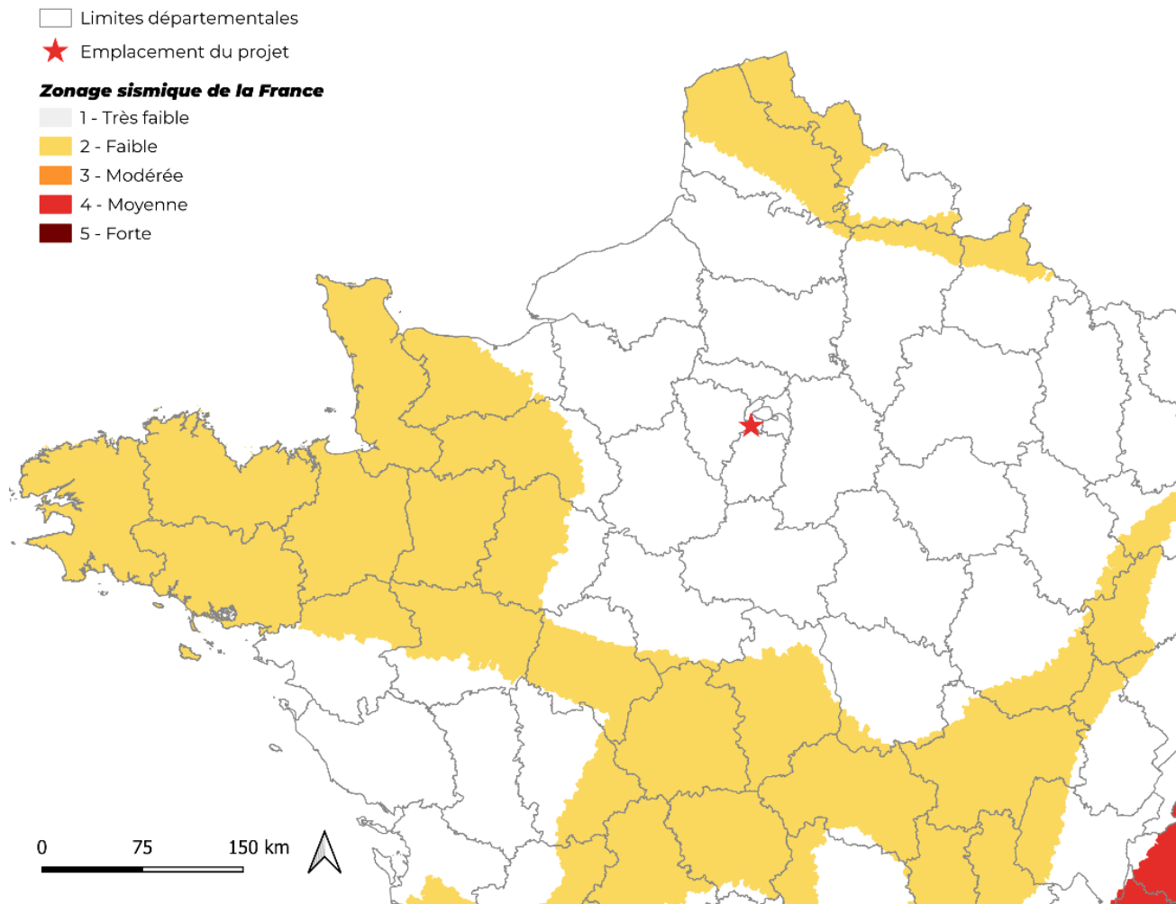
Zonage sismique de la France en vigueur (article D. 563-8-1 du Code de l'Environnement)
