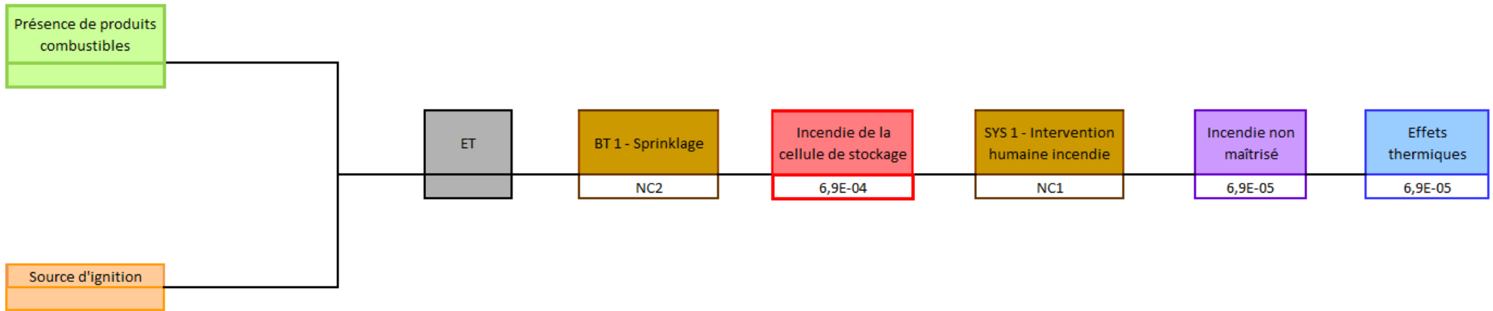
Nœud papillon 1 : Incendie d'une cellule de stockage de produits combustibles
