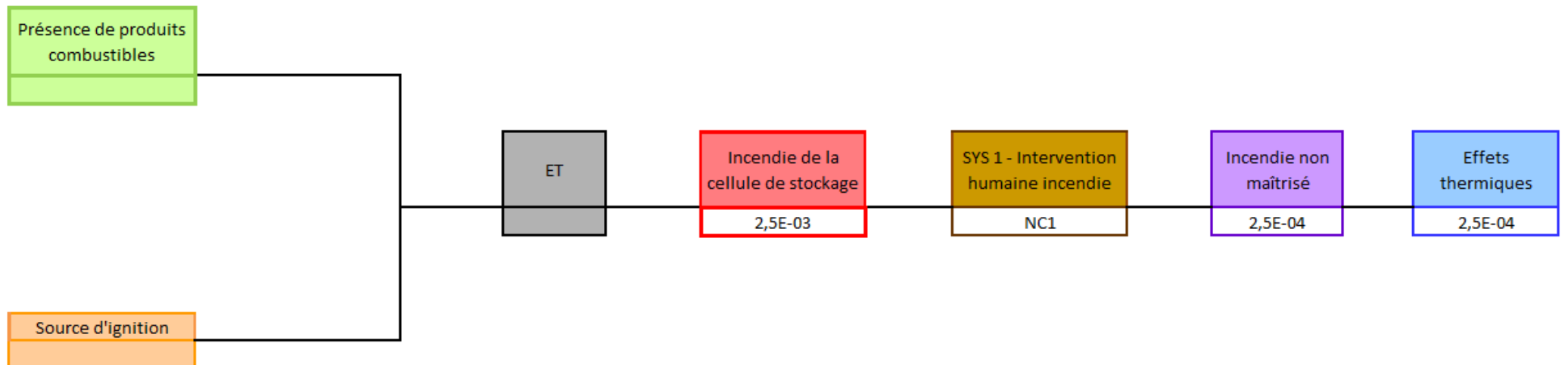
Nœud papillon 2 : Incendie d'une cellule de stockage frigorifique de produits combustibles
