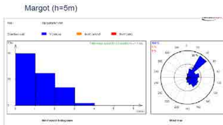
Rose des vents et vitesse des vents pour Margot (Source : étude SEURA)
