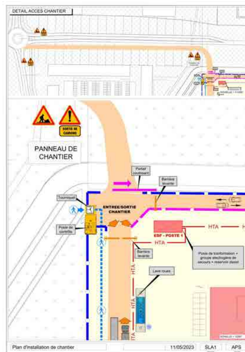
Figure 154 : Plan d'accès au chantier (source : Pizzarotti, 2023)
