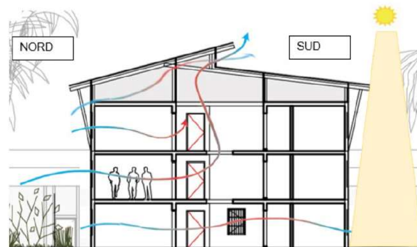
Figure 33 : Coupe bioclimatique schématique d'un quartier d'hébergement (source : Ingerop, 2024)
