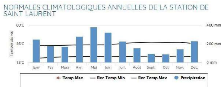
Figure 125 : Précipitations mensuelles moyennes à Saint-Laurent du Maroni Source : Météo-France Source : Météo-France
