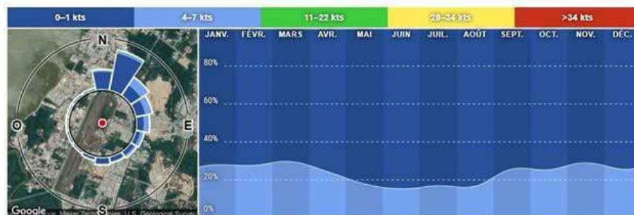
Figure 127 : Direction et répartition de la force du vent. Source : windfinder.com
