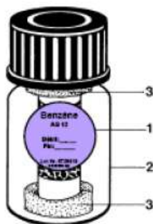
Figure 183 : Schéma d'un échantillonneur
