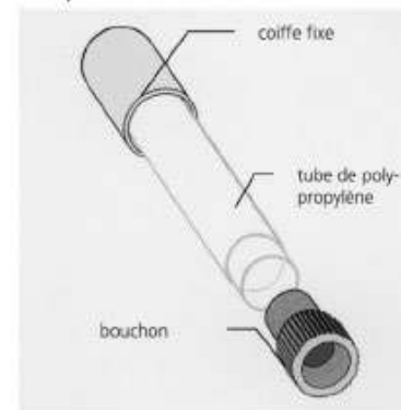
Figure 182 : Schéma d'un échantillonneur
