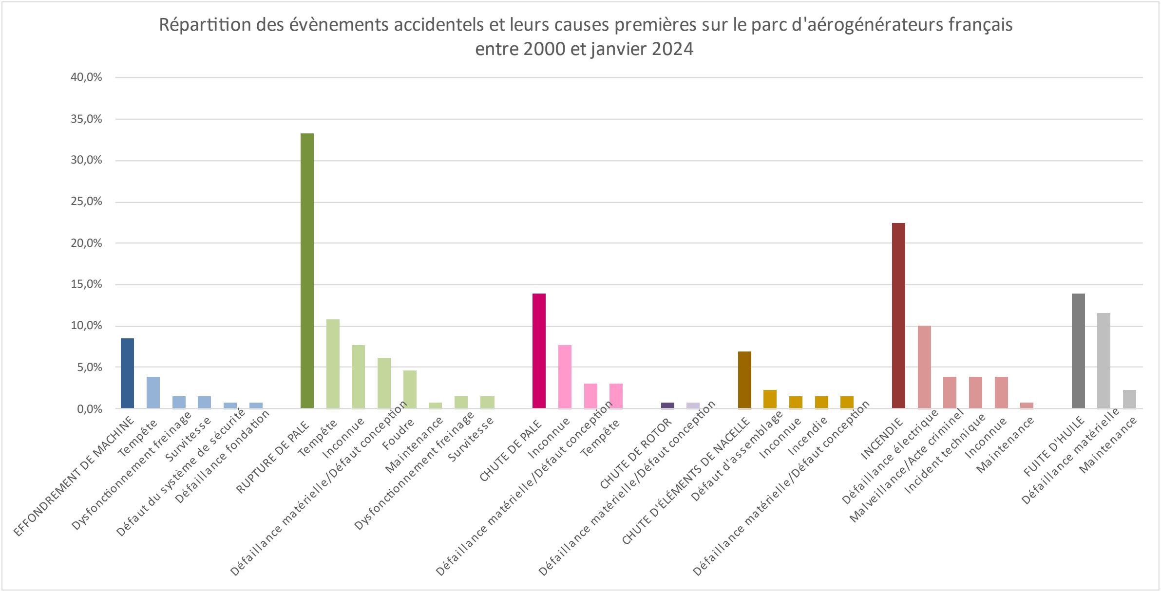
Figure 6 : Répartition des accidents et de leurs causes premières sur le parc éolien français entre 2000 et janvier 2024
