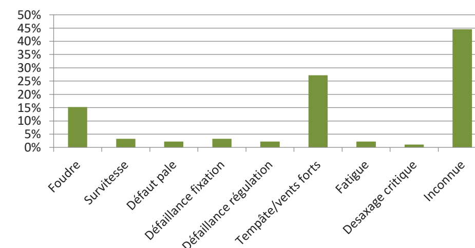
Figure 9 : Répartition des causes premières de rupture de pale dans les accidents à l'international entre 2000 et 2011
