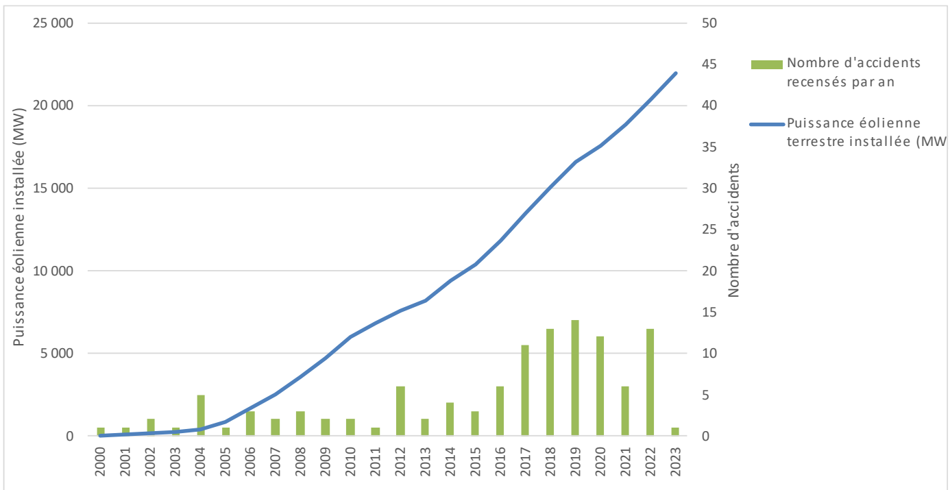
Figure 11 : Evolution du nombre d'accidents annuels en France et puissance éolienne installée depuis 2000
