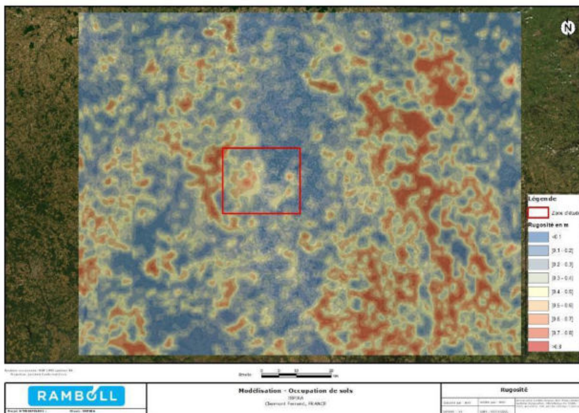
Figure 43 :Hauteur de rugosité utilisée dans le modèle ADMS
