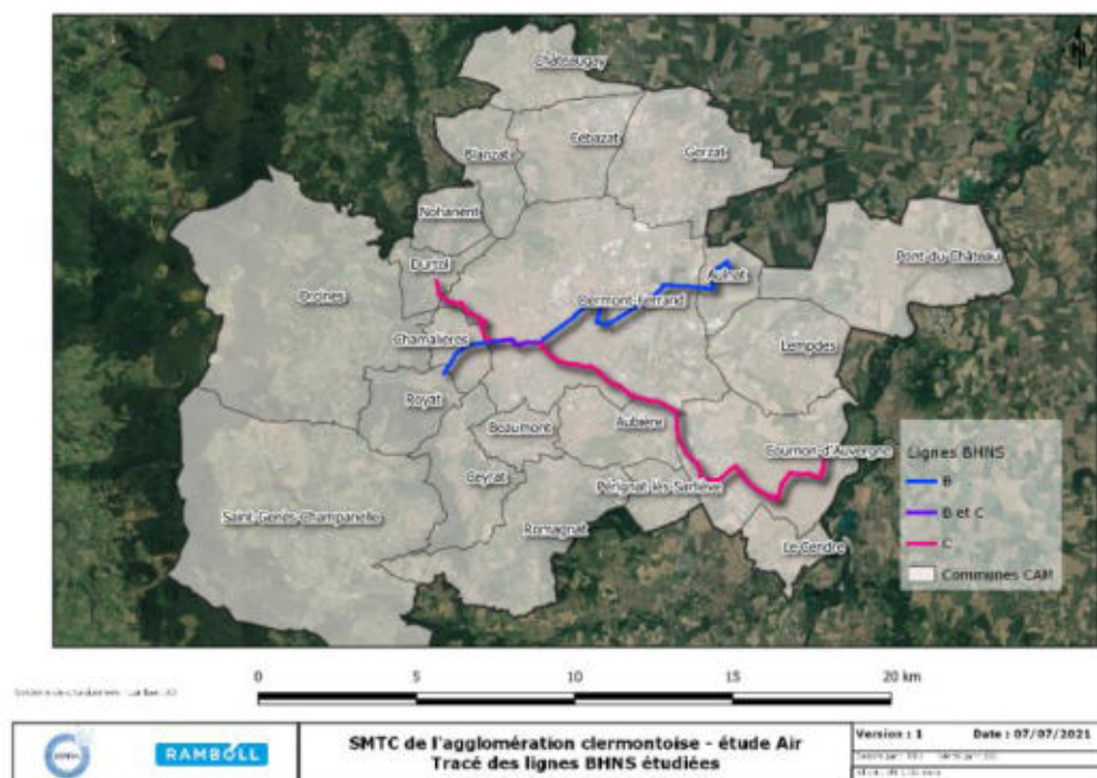
Figure 2 : Plan des hypothèses de tracé au stade de démarrage des études préliminaires (source SMTC-AC)
