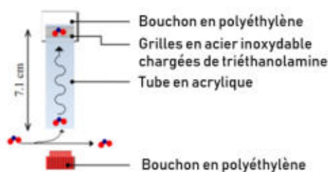
Figure 4 : Principe de l'échantillonneur passif Passam
