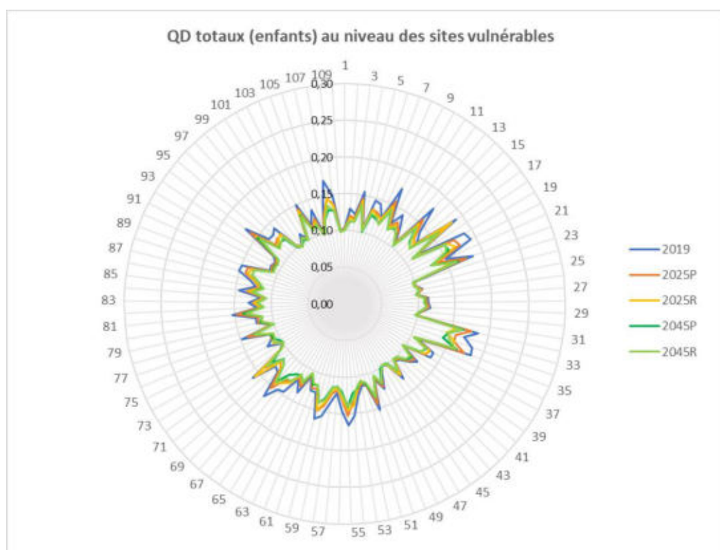
Figure 54 : Graphe des résultats des calculs de risque pour les effets chroniques à seuil (QD totaux enfant) au niveau des sites vulnérables
