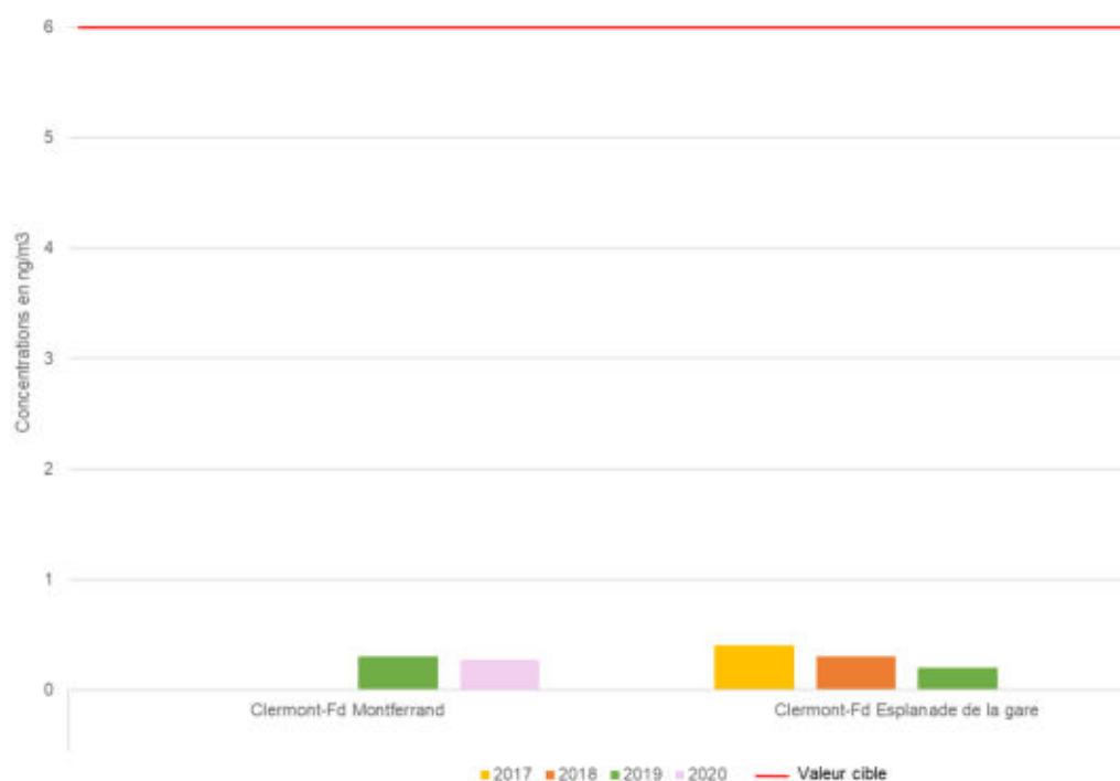
Figure 19 : Evolution des concentrations en moyenne annuelle en arsenic de 2017 à 2020 relevées à Clermont-Ferrand sur les stations d'Atmo AURA
