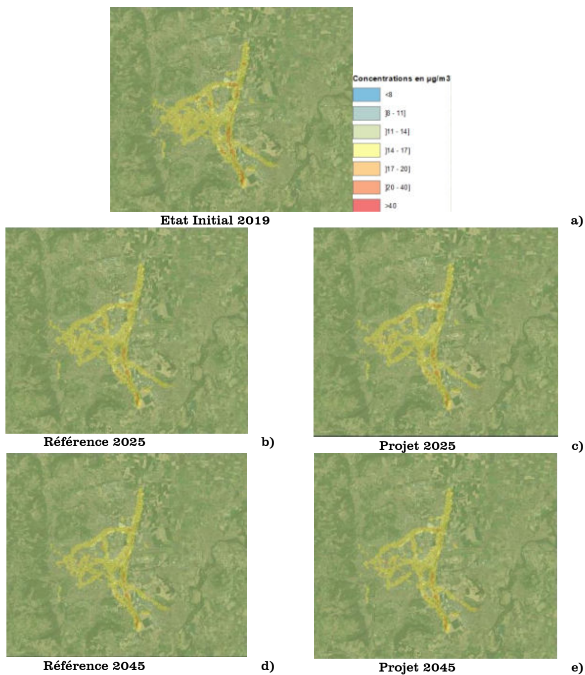
Figure 48 : Evolution des concentrations en \text{PM}_{10} sur l'ensemble de la zone d'étude - a)Etat Initial 2019, b) Référence 2025, c)Projet 2025, d)Référence 2045, e)Projet 2045
