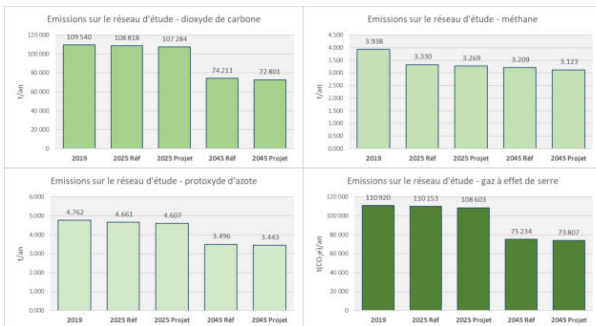
Figure 33 : Emissions en gaz à effet de serre selon le scénario sur le réseau d'étude
