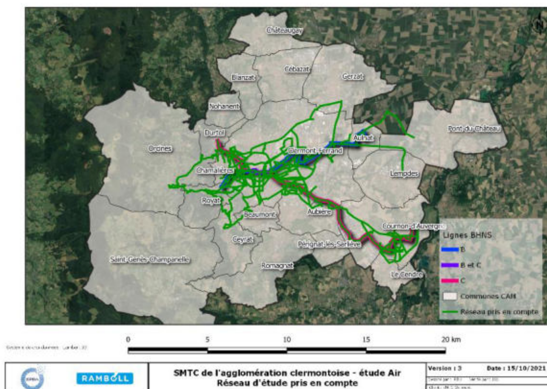
Figure 27 : Réseau d'étude pris en compte
