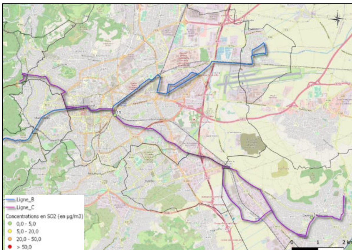
Figure 25 : Cartographie des concentrations moyennes en SO_2 sur les quatre campagnes de l'étude
