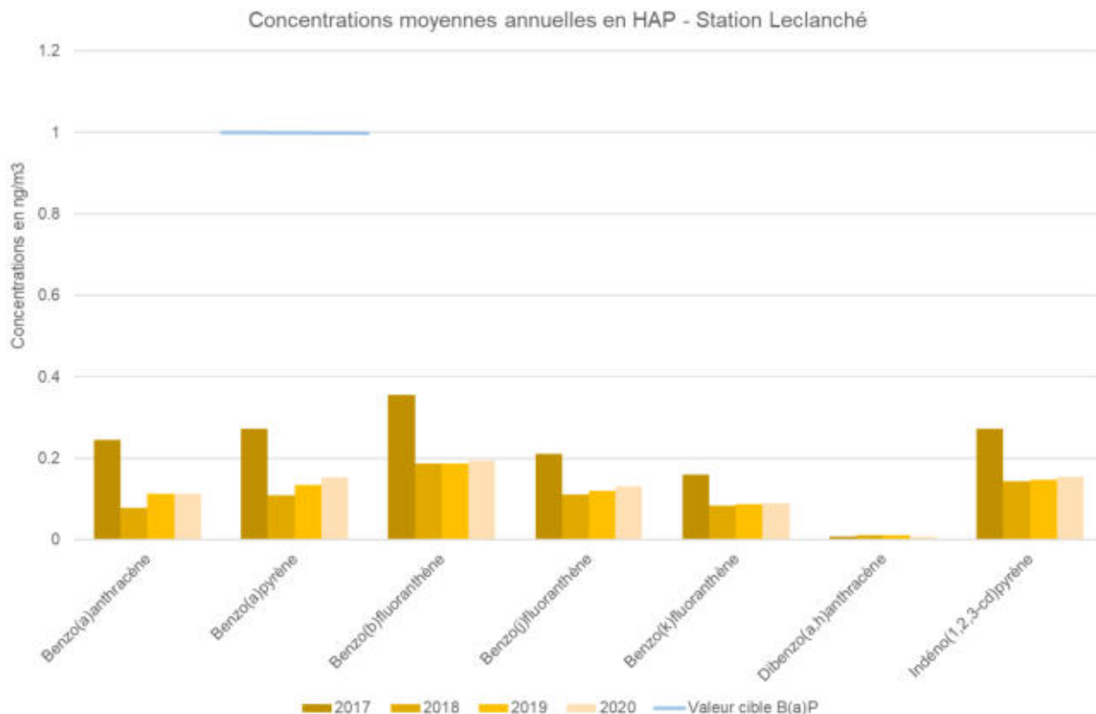
Figure 17 : Evolution des concentrations en moyenne annuelle en HAP de 2017 à 2020 relevées à Clermont-Ferrand sur la station Leclanché
