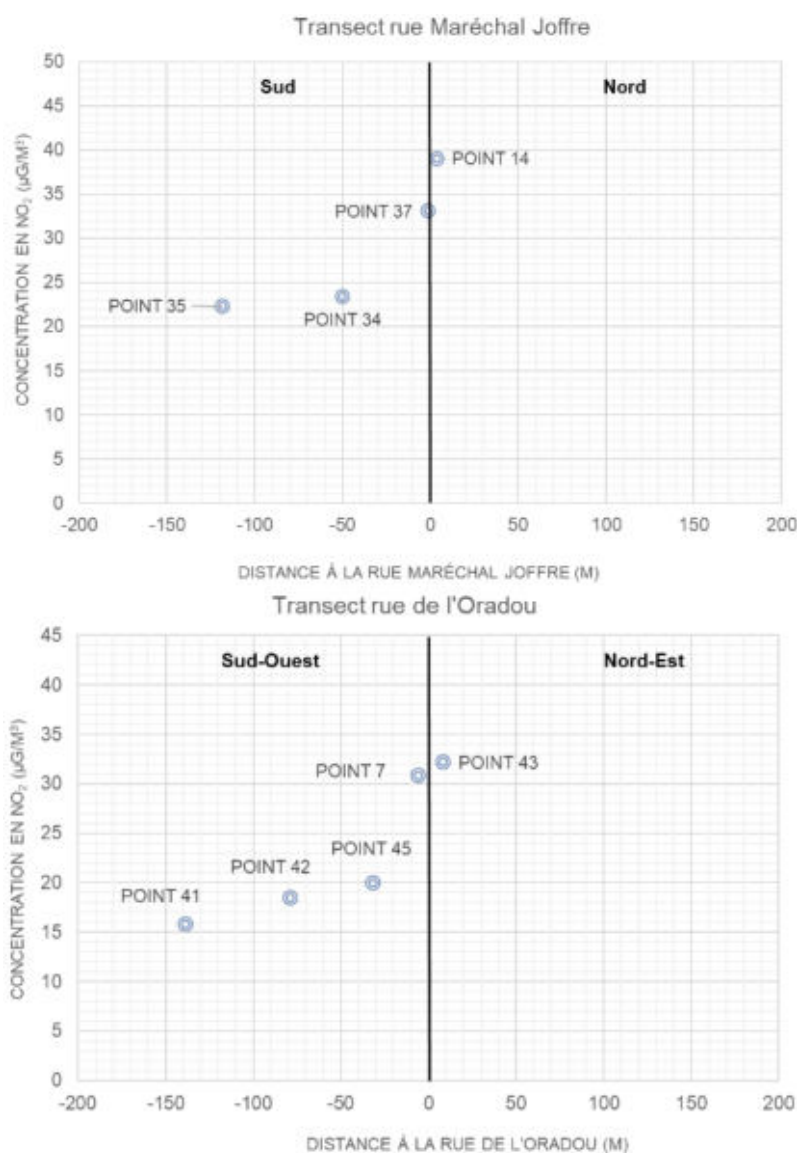
Figure 22 : Concentrations en \text{NO}_2 relevées sur les transects rue du Maréchal Joffre et rue de l'Oradou en moyenne sur les quatre campagnes de l'étude
