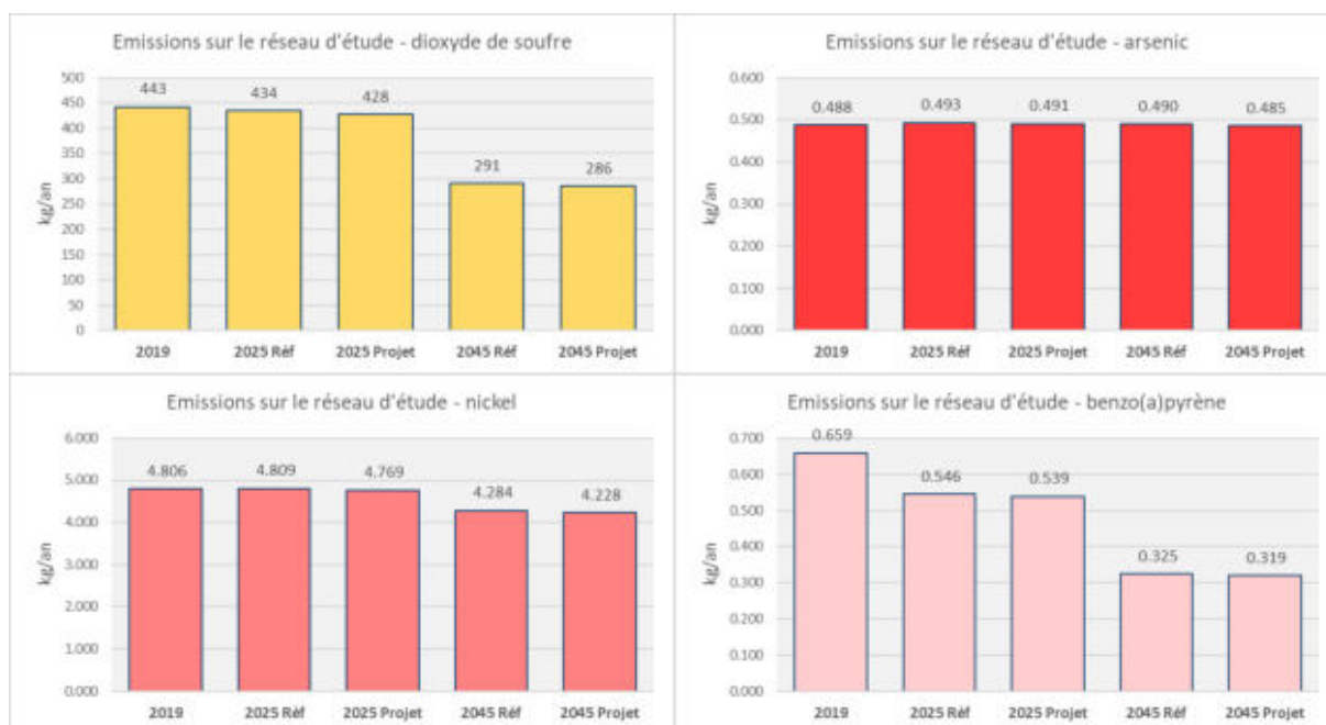
Figure 32 : Emissions en polluants selon le scénario sur le réseau d'étude
