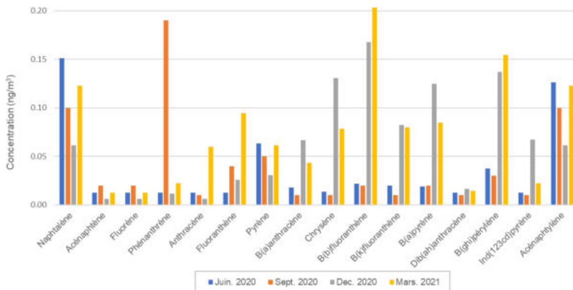
Figure 26 : Comparaison des concentrations en HAP mesurées lors des différentes campagnes de juin, septembre, décembre 2020 et mars 2021
