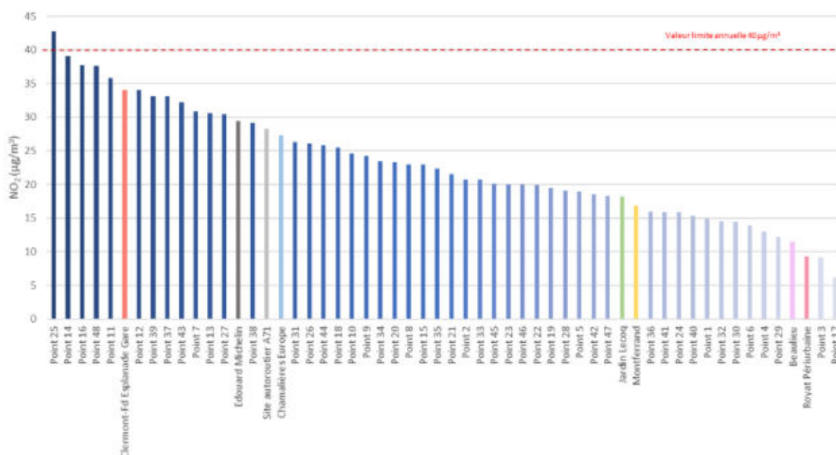
Figure 23 : Concentrations en \text{NO}_2 relevées sur les différents points de mesure et aux stations d'Atmo AURA moyennées sur les quatre campagnes de l'étude
