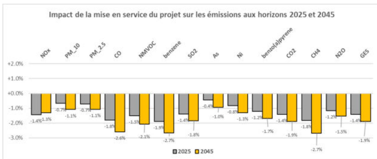
Figure 35 : Impact de la mise en service du projet sur les émissions aux horizons 2025 et 2045 selon le scénario sur le réseau d'étude
