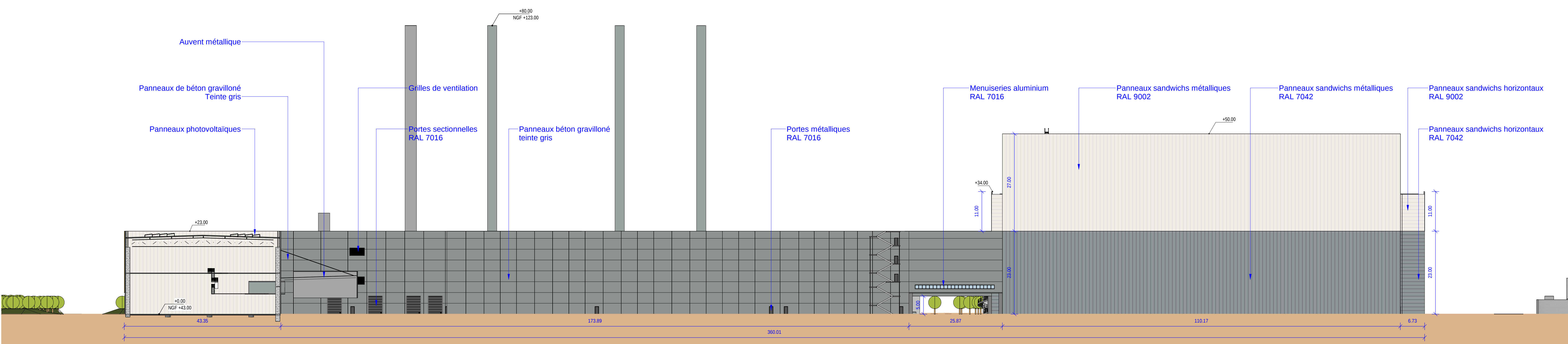
ELEVATION NORD - 1: 500
